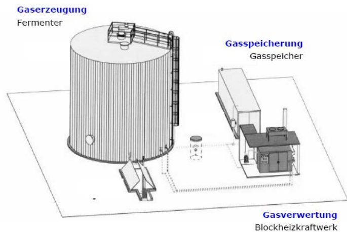
Bild 2: Schematische Darstellung der Gaserzeugung
